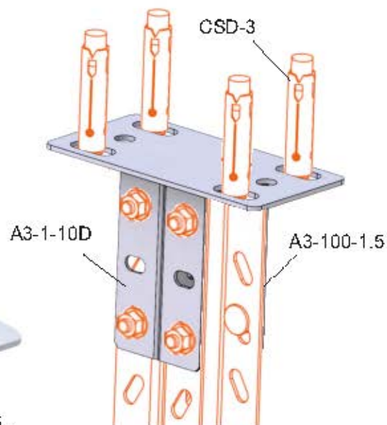
A3-1-10D Примерна връзка
