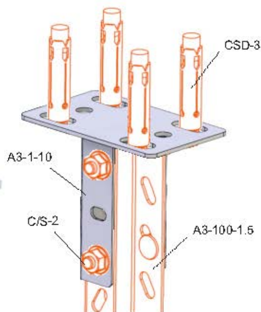
A3-1-10 Примерна връзка
