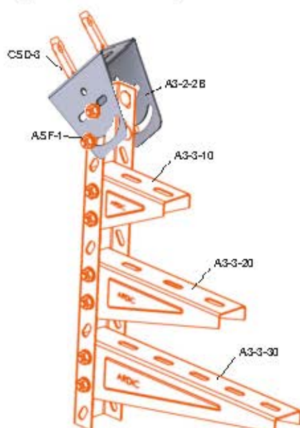
A3-2-2B Примерна връзка
