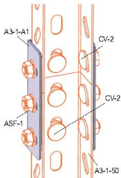
A3-1-A1 Примерна връзка
