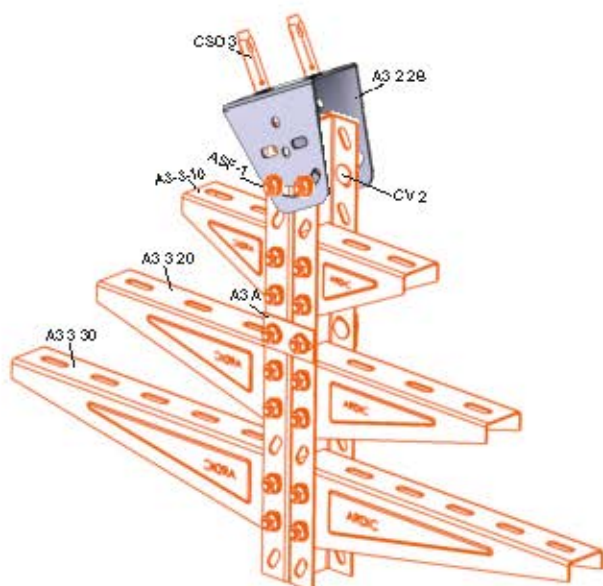
A3-2-2B Примерна връзка
