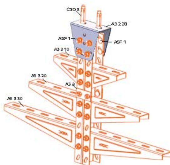
A3-2-2B Примерна връзка
