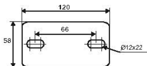
Детайли за базов отвор
