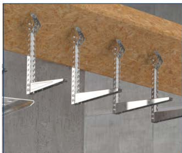
Приложение за носещи скоби
